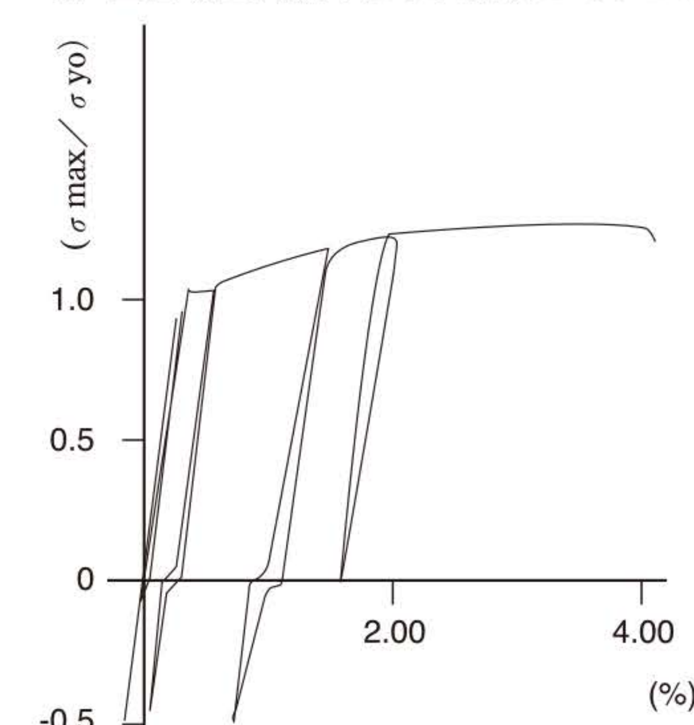
弾・塑性域正負繰返し試験 (SD490 D41)
